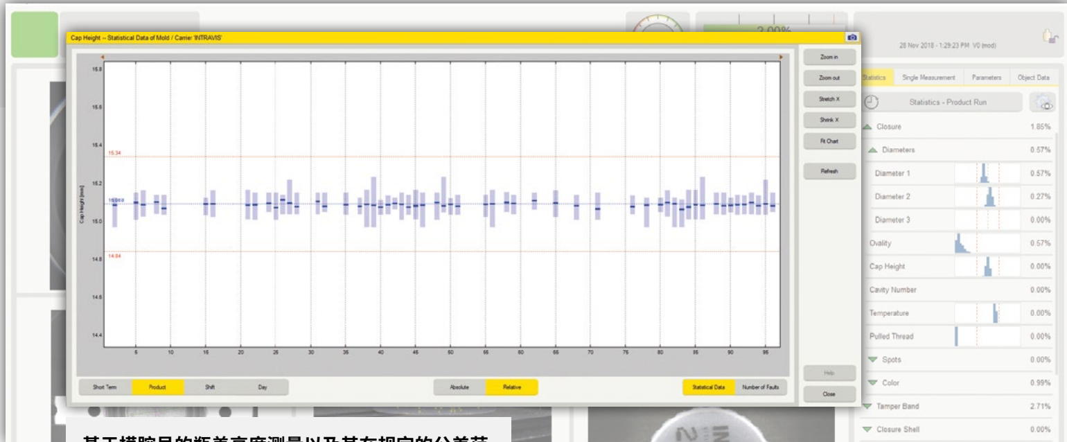
基于模腔号的瓶盖高度测量以及其在规定的公差范围内的散布
