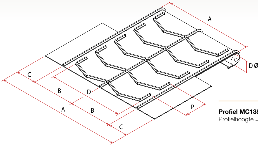
Profiel MC1380
