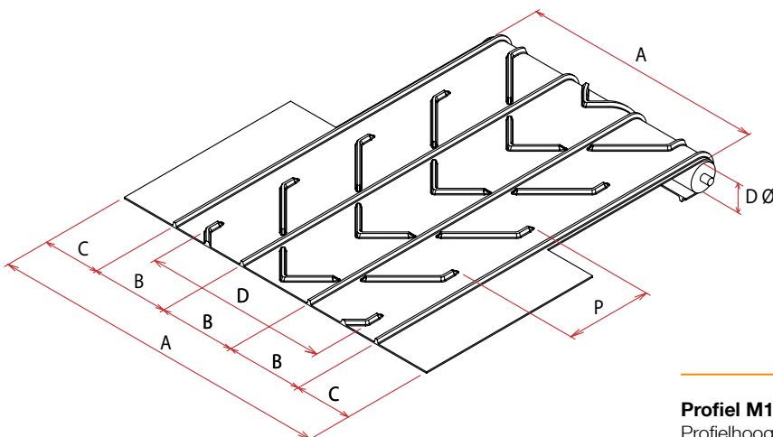
Profiel M1335
